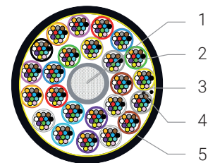
MCD1520 288 Fasern 24 Tubes à 12 Fasern
