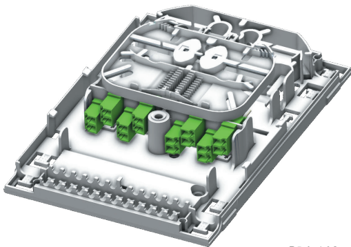
PBA-16C mit 8 LC/APC Duplex Kupplungen
