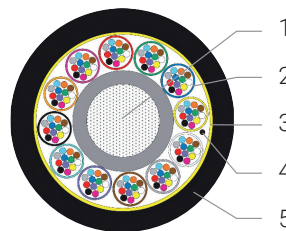
MCD1520 144 Fasern 12 Tubes à 12 Fasern
