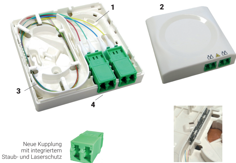
Ablage für 4x Crimpspleißschutz
